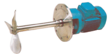
Agitator "LMR"
